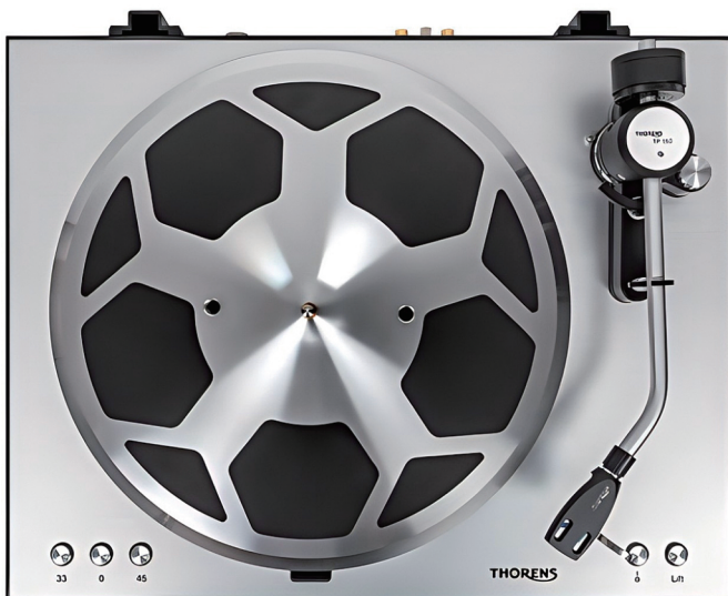
▲ 转盘经过厂方的精密计算，加入阻尼物料，除了能够承托唱片之外，还能吸收转盘工作时的振动
